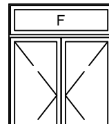
Puerta calle exterior 2 hojas con fijo superior
